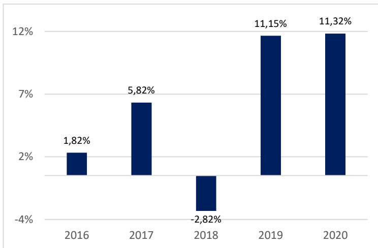
Performances Annuelles de Varenne Valeur part I-EUR
